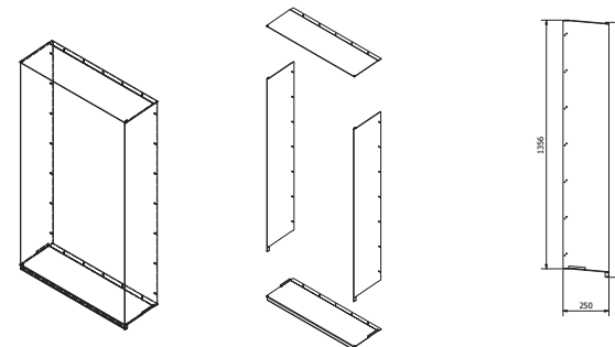
FZB503 CADRE COMPLET
